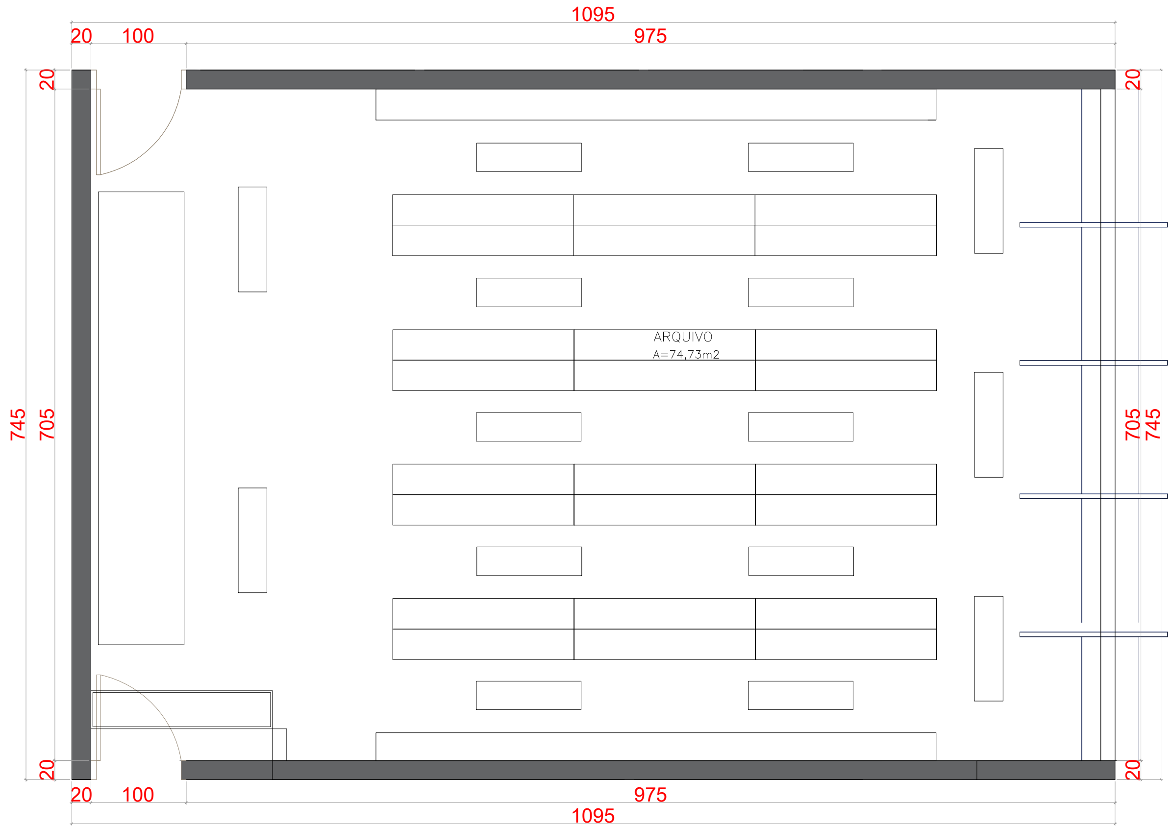
PLANTA BAIXA - ARQUIVO MÉDICO SEM ESCALA .....
