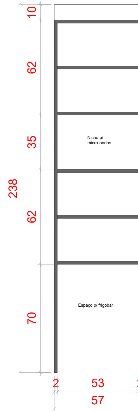
Vista Interna
