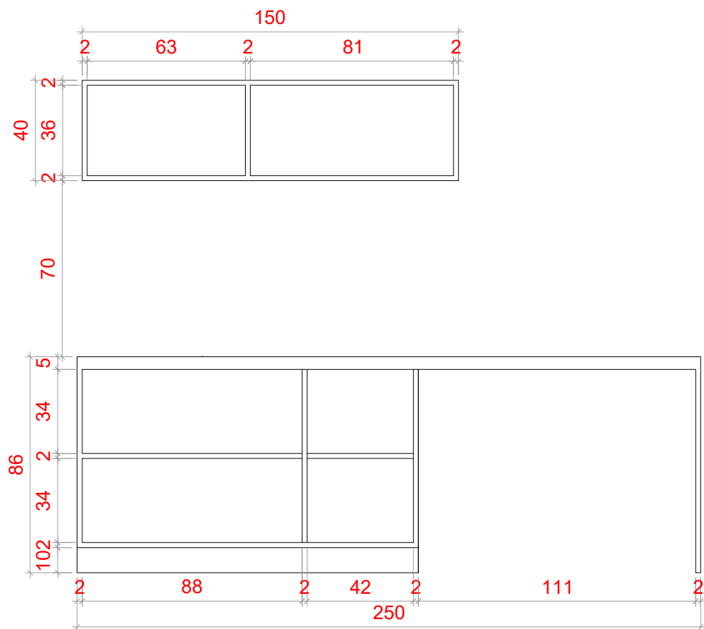
Vista Interna
