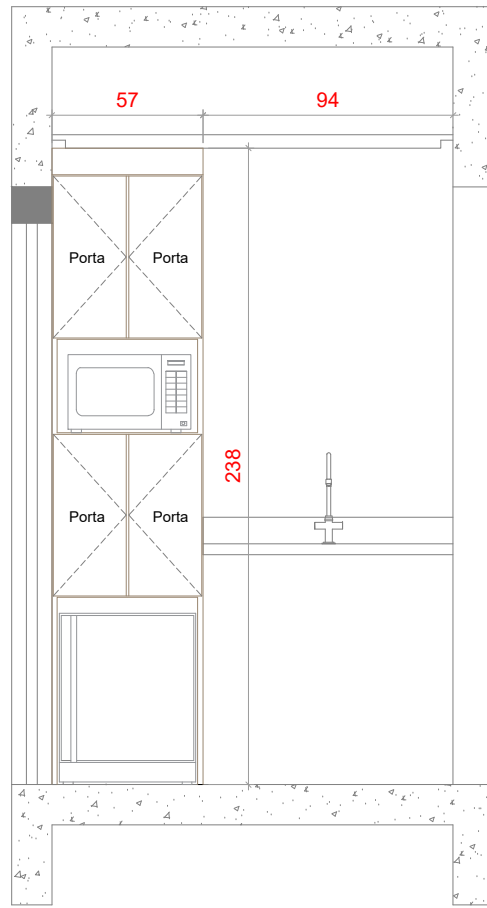
Corte
