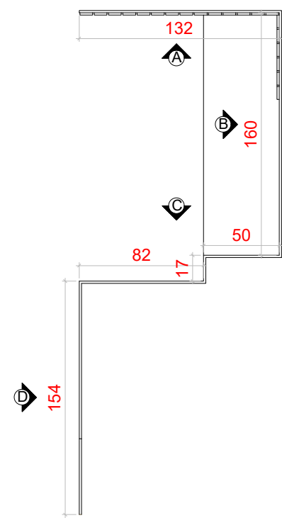
VISTA SUPERIOR - em planta SEM ESCALA .....
