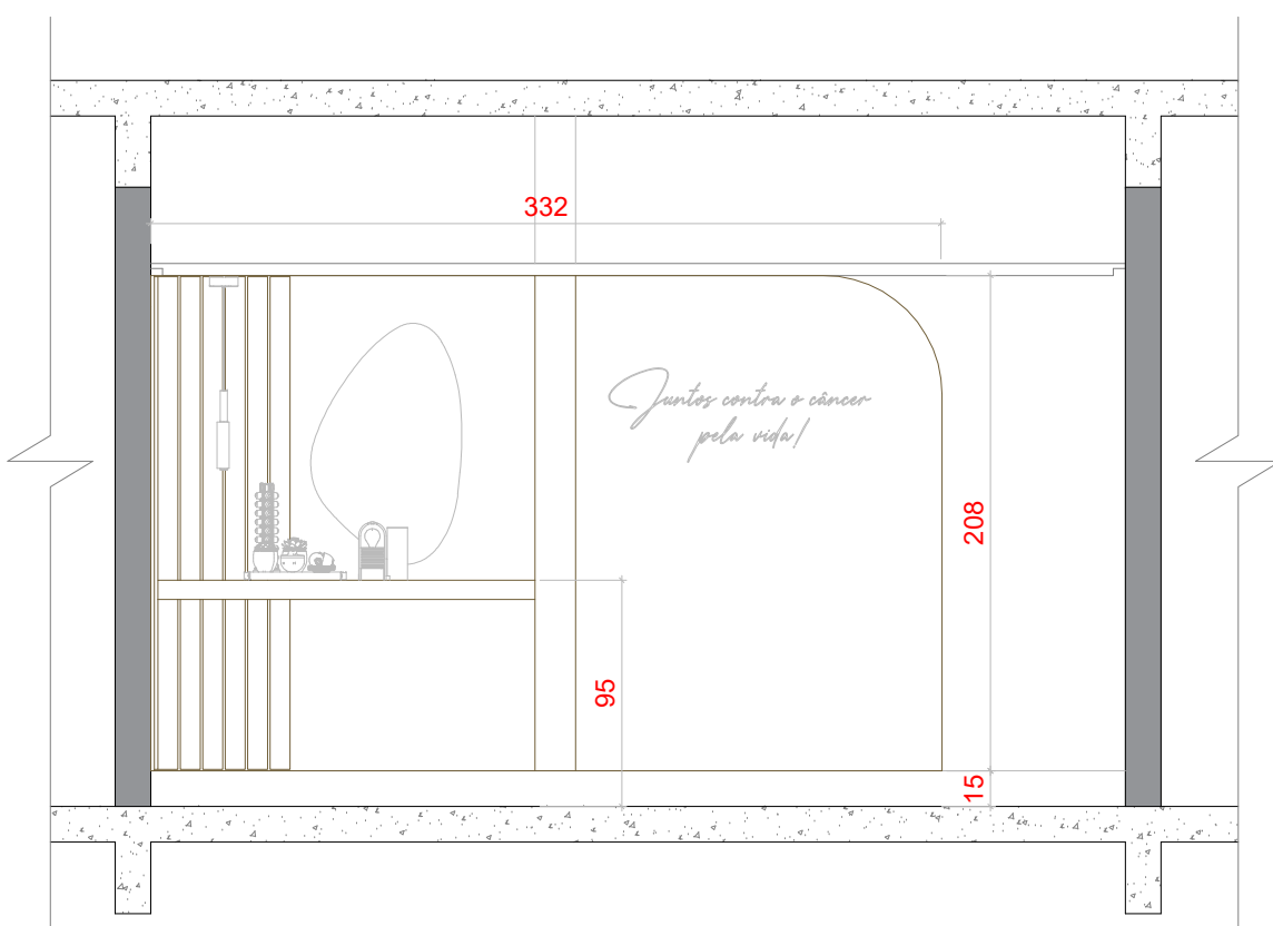
VISTA SEM ESCALA .....
