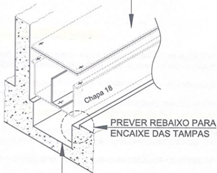
DET. 04 - CANALETAS EMBUTIDAS NO PISO 20x15cm - VISTA EM PERSPECTIVA, LATERAL E PLANTA Sem escala
