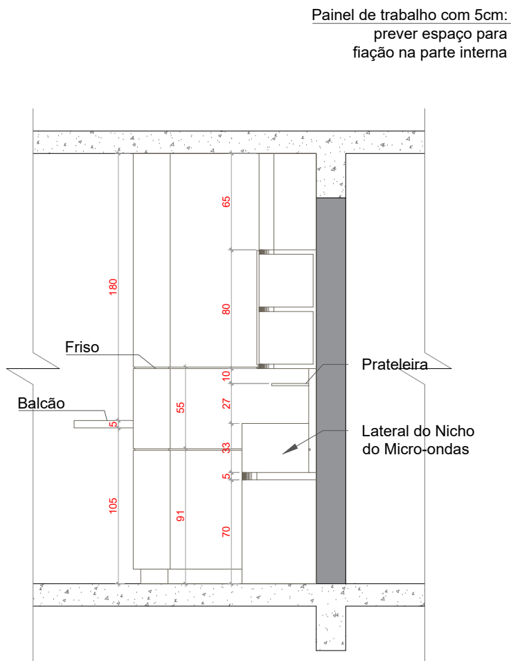
Vista Lateral
