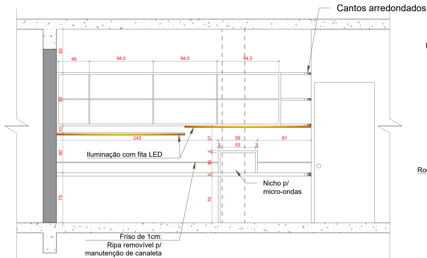
Vista Interna
