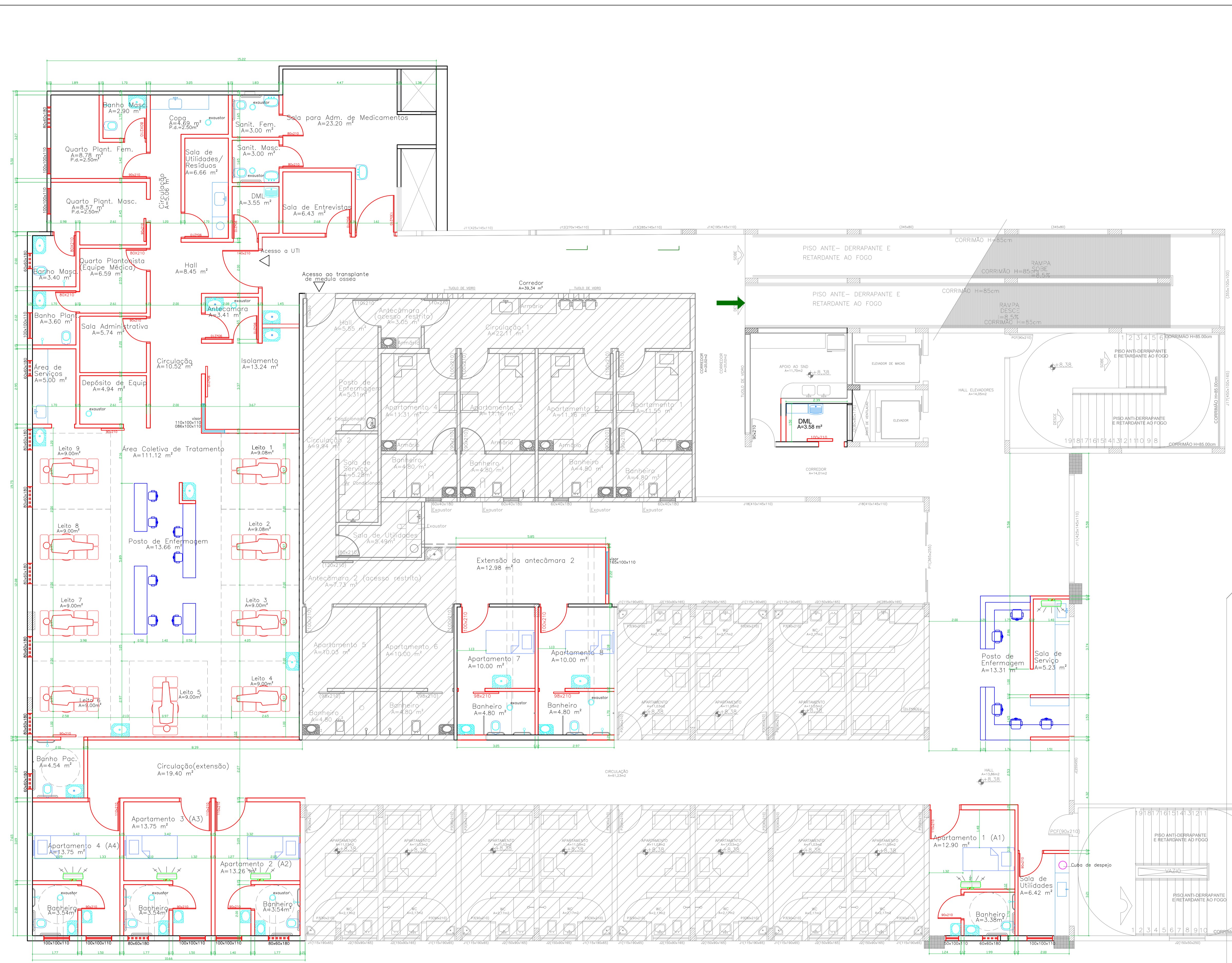
Planta Baixa do 2º Pavimento Reforma Cotas- UTI, transplante de médula óssea (2 leitos), apartamentos e apoio Esc: 1/75
